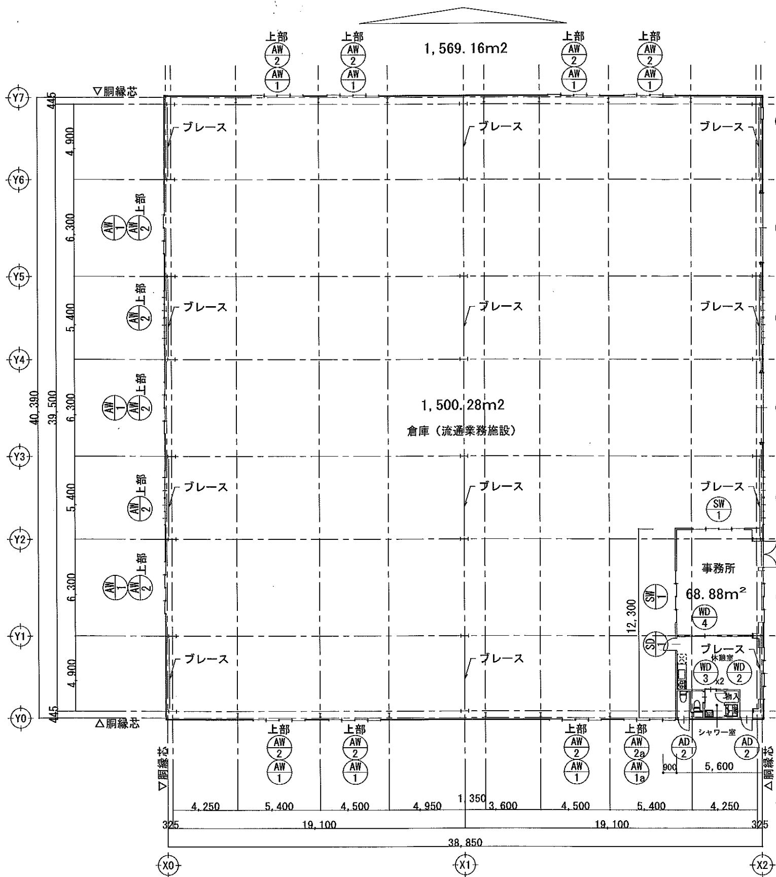
平面図 S=1/250
